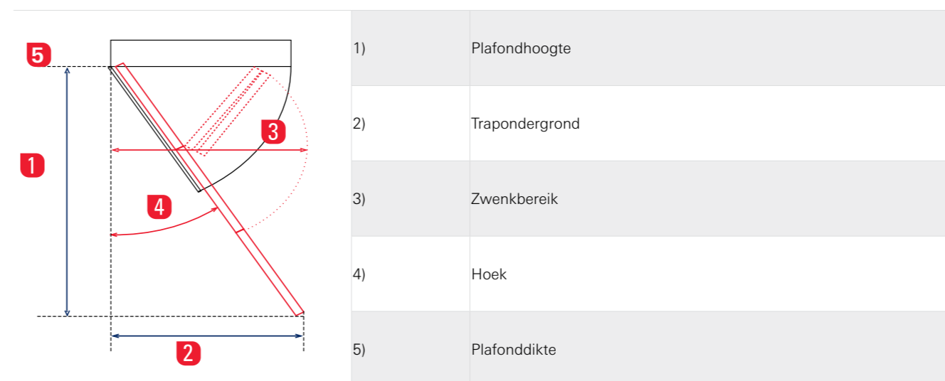
Technische schets 3-delige trap
