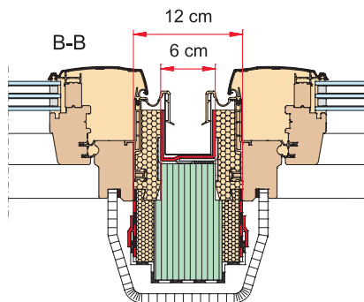
Combinatie met koppelspar en Roto binnenafwerking voor meer licht en meer vrije ruimte bovenin
