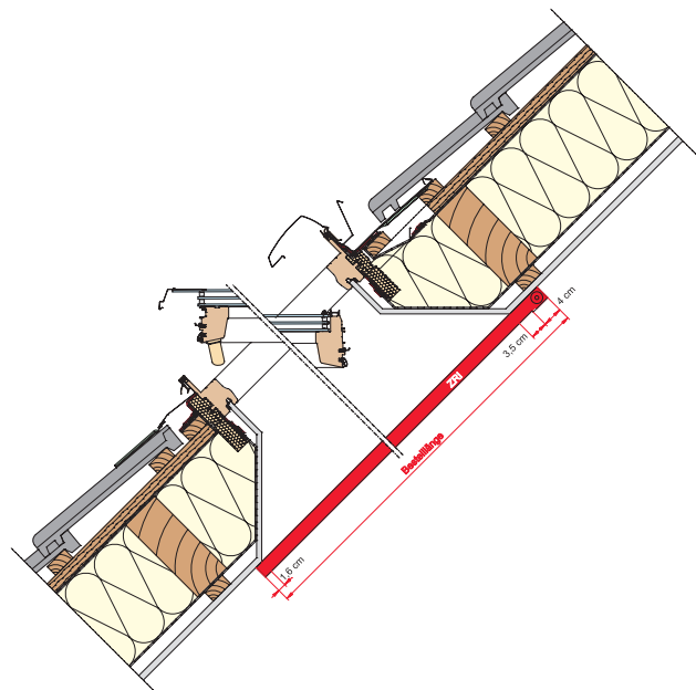
Afb. 7: Bestellengte voor insectenhor op de muur/wand ZRI M W; binnenwerkse breedte binnenafwerking + 9,1 cm.
