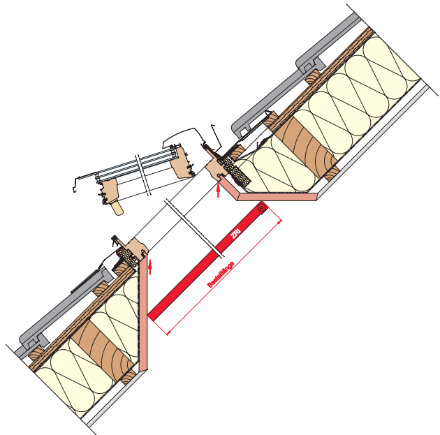
Afb. 5: Designo R8 uitzet-tuimelraam insectenhor in het kozijn ZRI M L, vanwege een schuine of naar buiten staande binnenafwerking.
