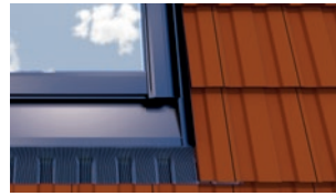
RotoQ Gootstukken verdiept geplaatst ETW Qx Dakpan verlaagd
