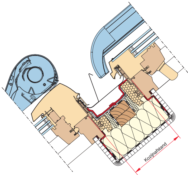
Boven elkaar R6/R8: kozijnafstand 140 mm
