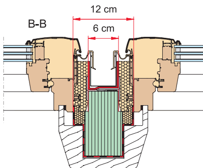
Combinatie met koppelspar en massieve houten bekleding voor meer licht en meer vrije ruimte bovenin
