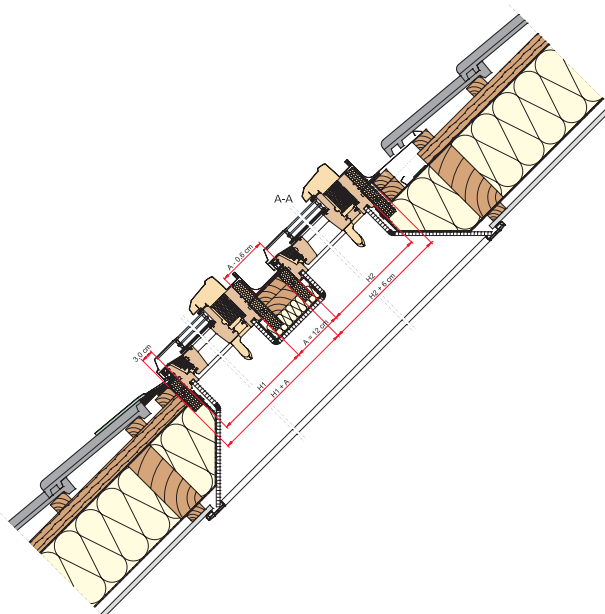
Naast elkaar R6/R8: UBL-breedte bij 140 mm kozijnafstand
