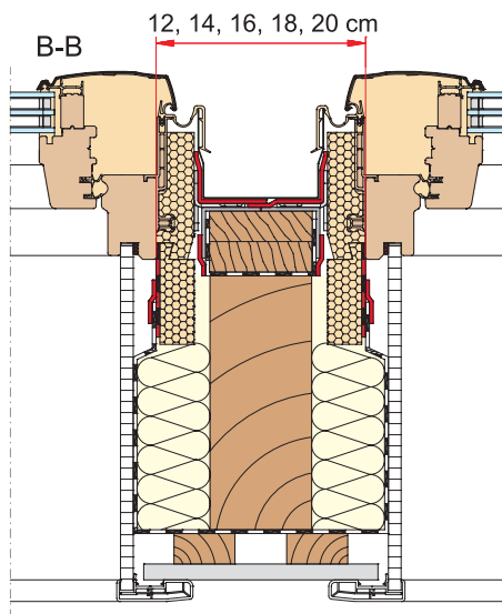
Combinatie naast elkaar met een kozijnafstand vanaf 120 mm
