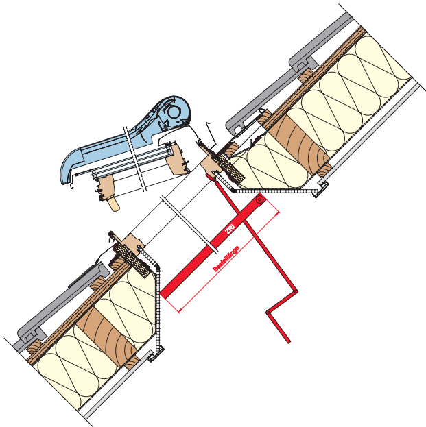
Afb. 4: Designo R8 uitzet-tuimelraam met handmatig buitenrolluik en insectenhor in het kozijn ZRI M L, zodat de kruk kan worden aangebracht.
