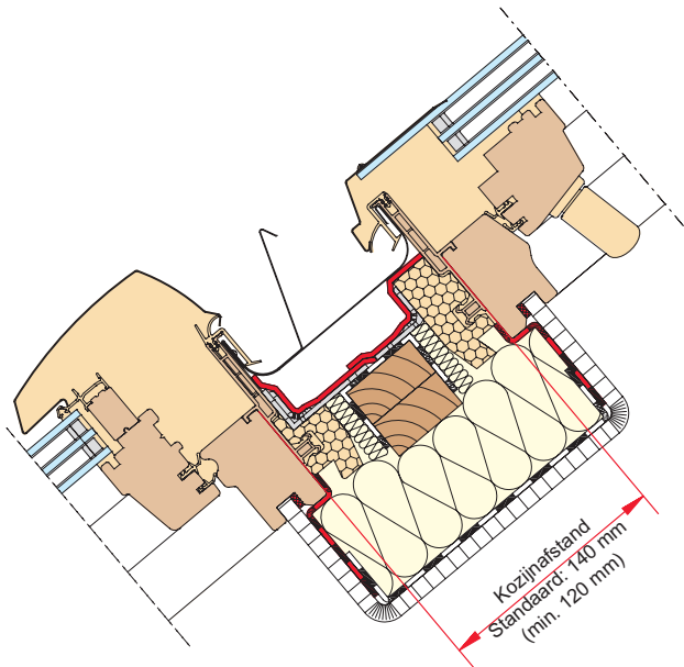
Boven elkaar R6/R8: kozijnafstand 140 mm
