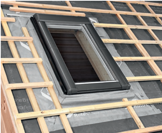
Het extern aansluitmanchet ingebouwd
