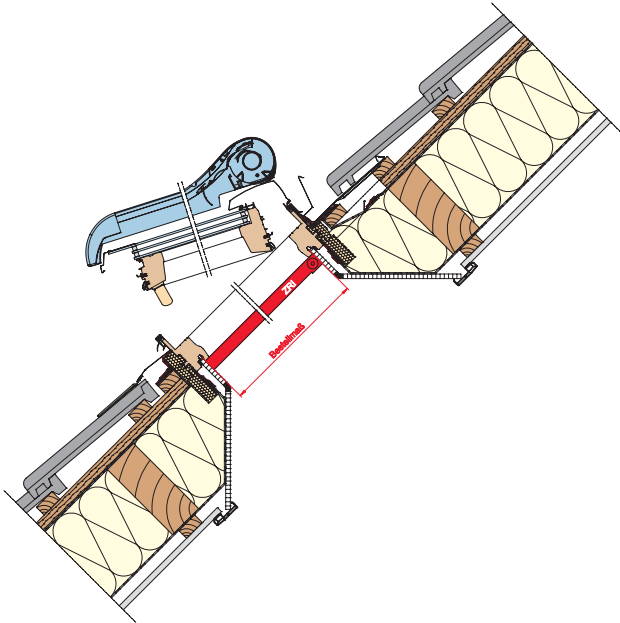
Afb. 1: Designo R8 uitzet-tuimelraam met insectenhor aan het raamkozijn ZRI M.B
