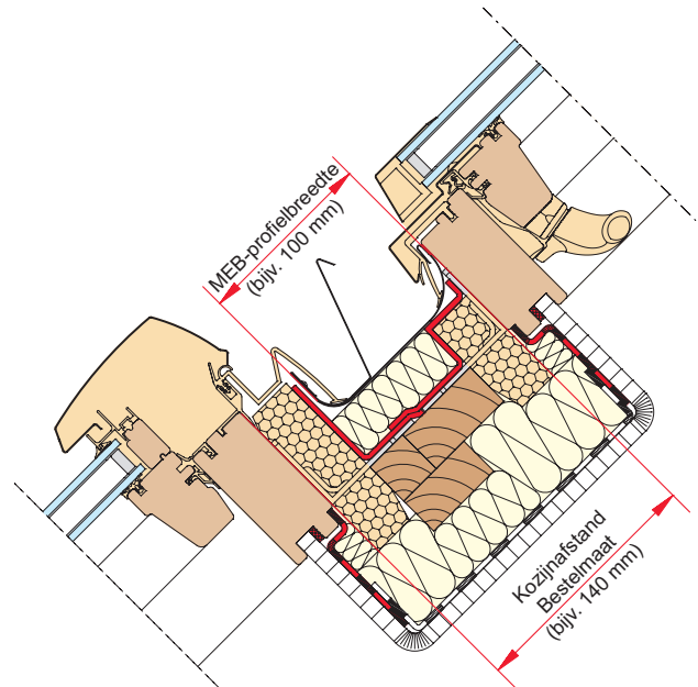
Boven elkaar R7: MEB-breedte bij 140 mm kozijnafstand
