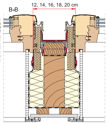
Standaard combinatie met spar op plaats van montage, minder licht en minder vrije ruimte bovenin
