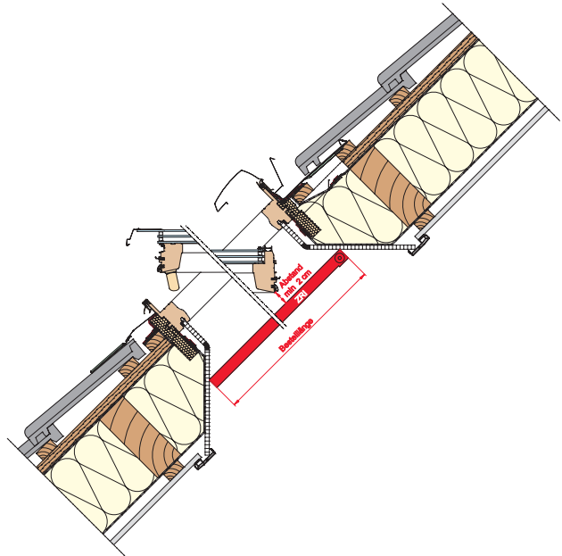
Afb. 3: Bestellengte voor insectenhor in het kozijn ZRI M L; min. 2 cm afstand tot het geopende vleugelkozijn is noodzakelijk
